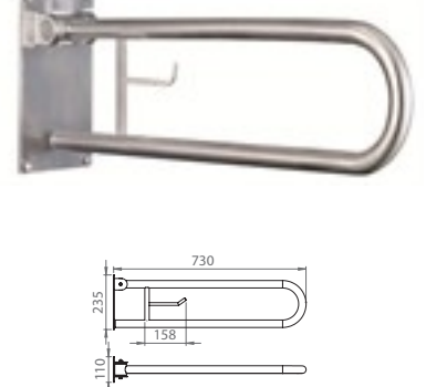
Klozet Tutunma Bari Kağıtlıklı
