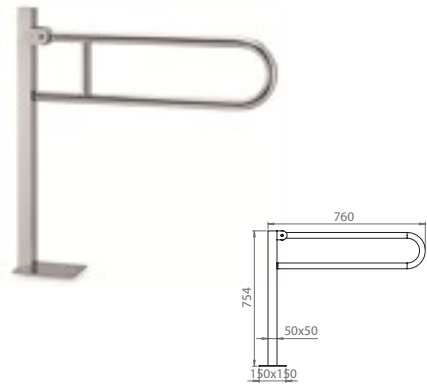
Ayaklı Mafsallı Engelli Tutunma Bari
