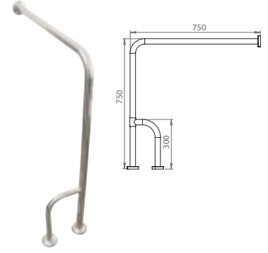
Engelli Tutunma Bari
