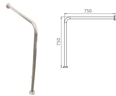
Engelli Tutunma Bari
