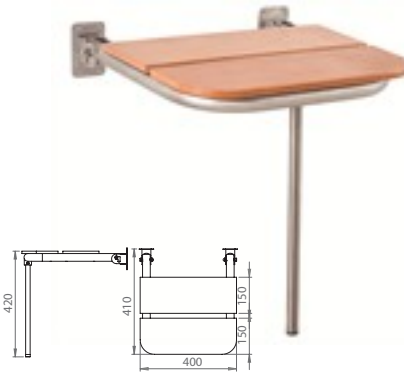
Engelli Duş Oturağı Ahşap
