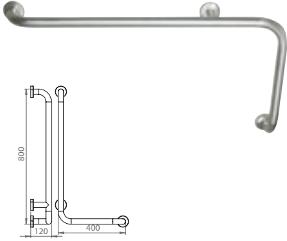
Engelli Tutunma Bari
