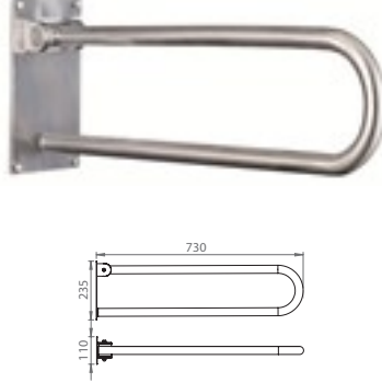
Klozet Tutunma Bari
